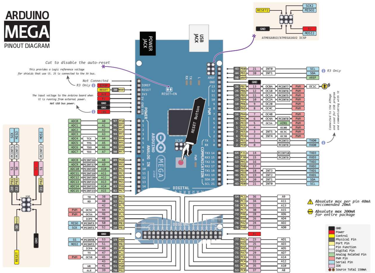
Abbildung 7.3. Arduino Mega
