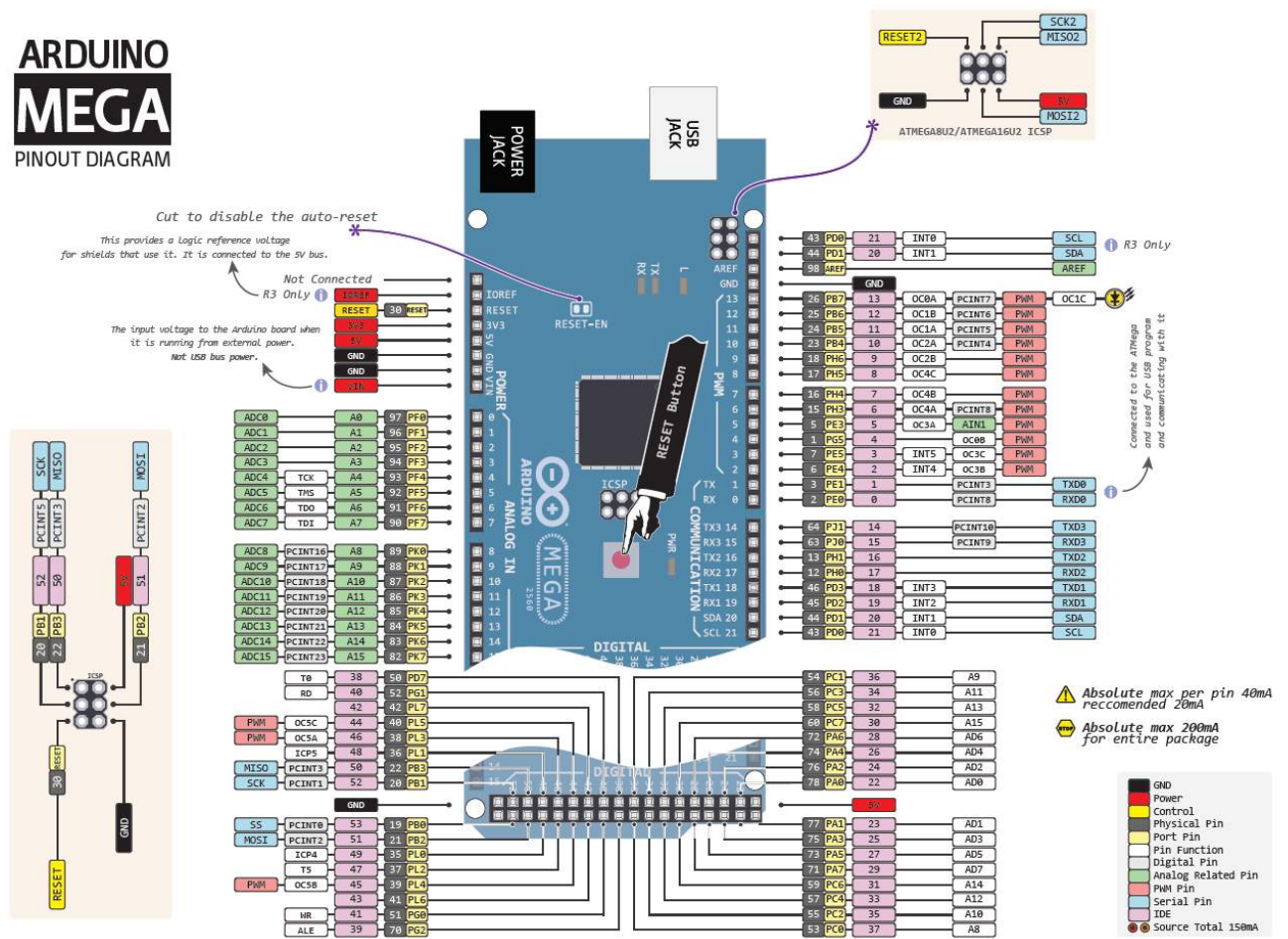
Abbildung 7.3. Arduino Mega
